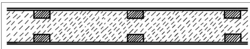
Rys. 10. Przekrój fundamentu betonowego (rys. J. Tajchman)
